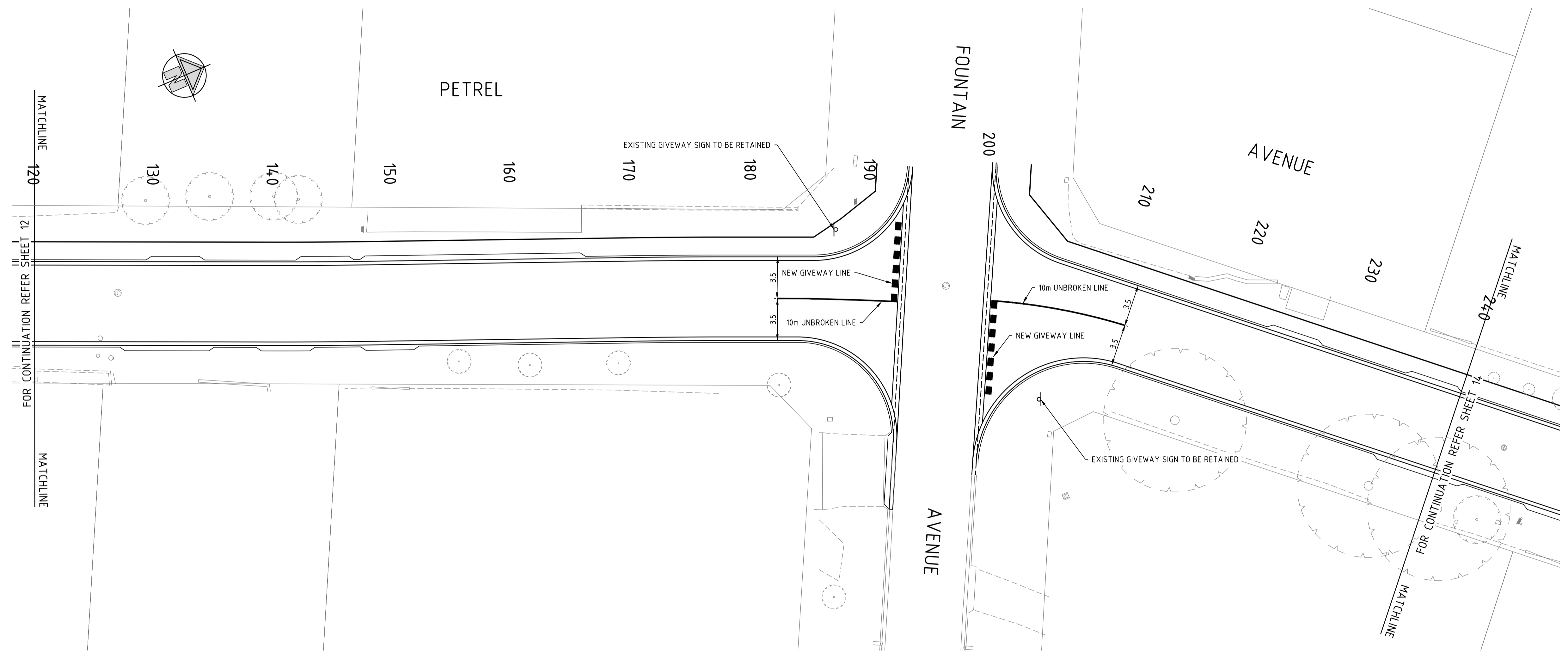
PLAN SCALE: 1:200
