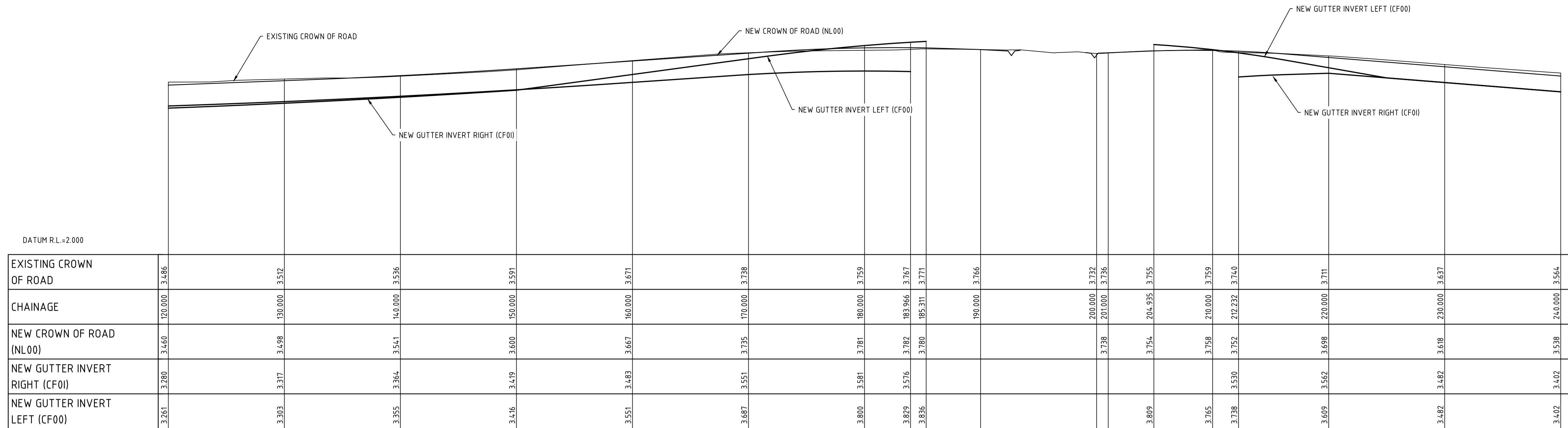
LONGITUDINAL SECTION SCALE: H - 1:200, V - 1:20
