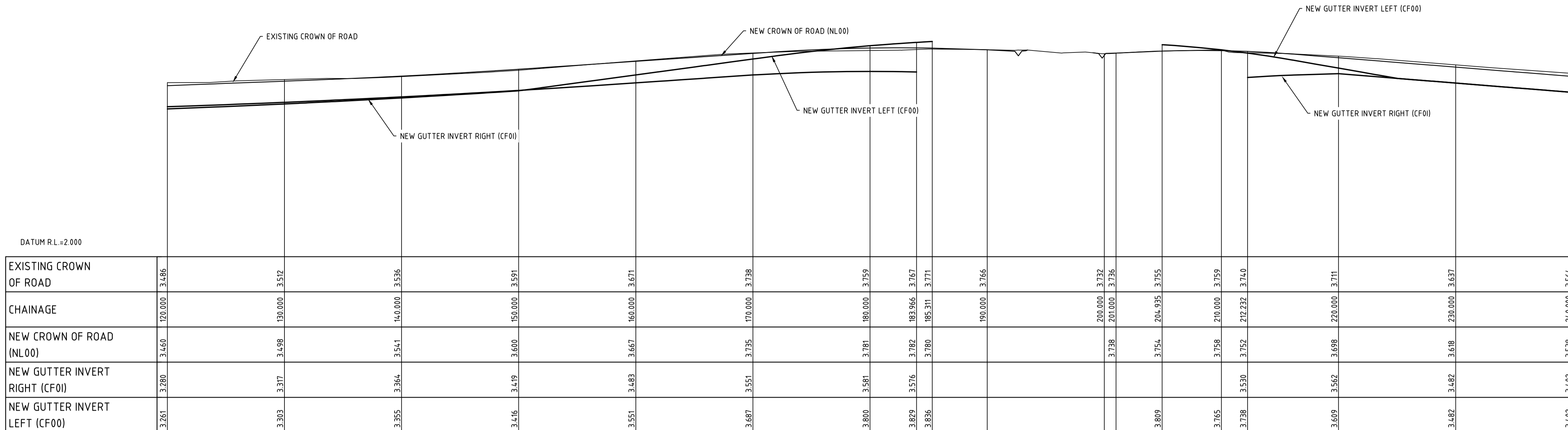
LONGITUDINAL SECTION SCALE: H - 1: 200, V - 1: 20
