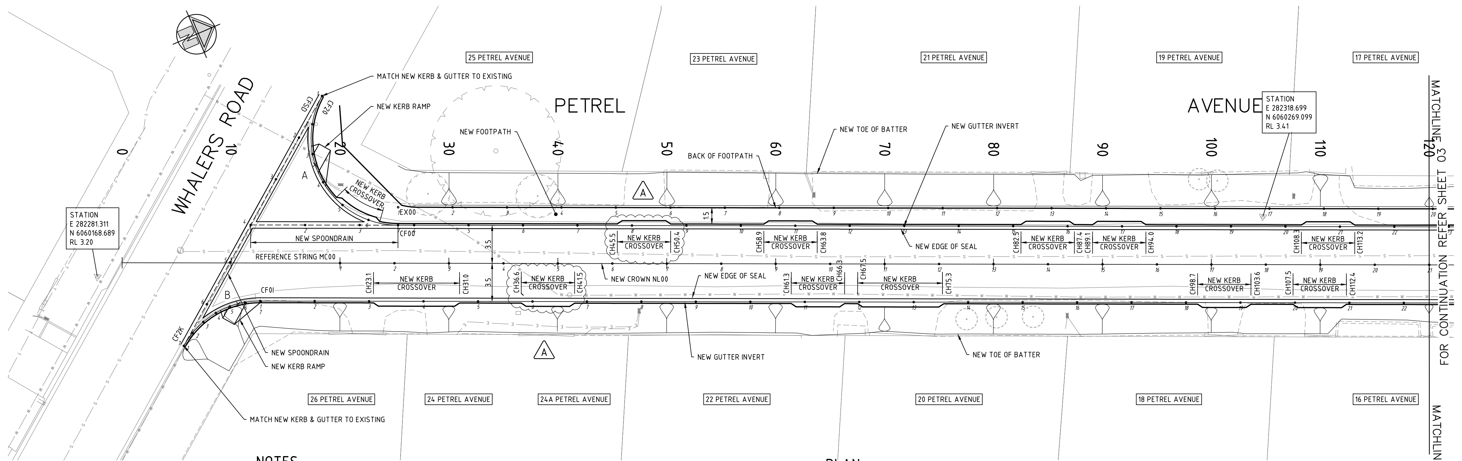
PLAN SCALE: 1:200
