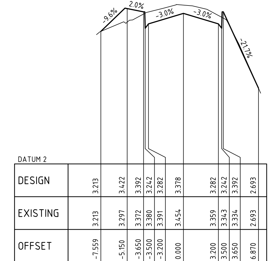
CHAINAGE 260.000
