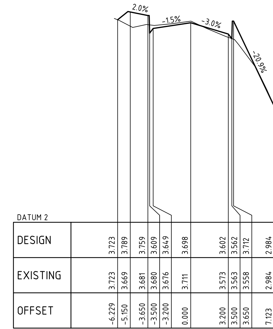
CHAINAGE 220.000
