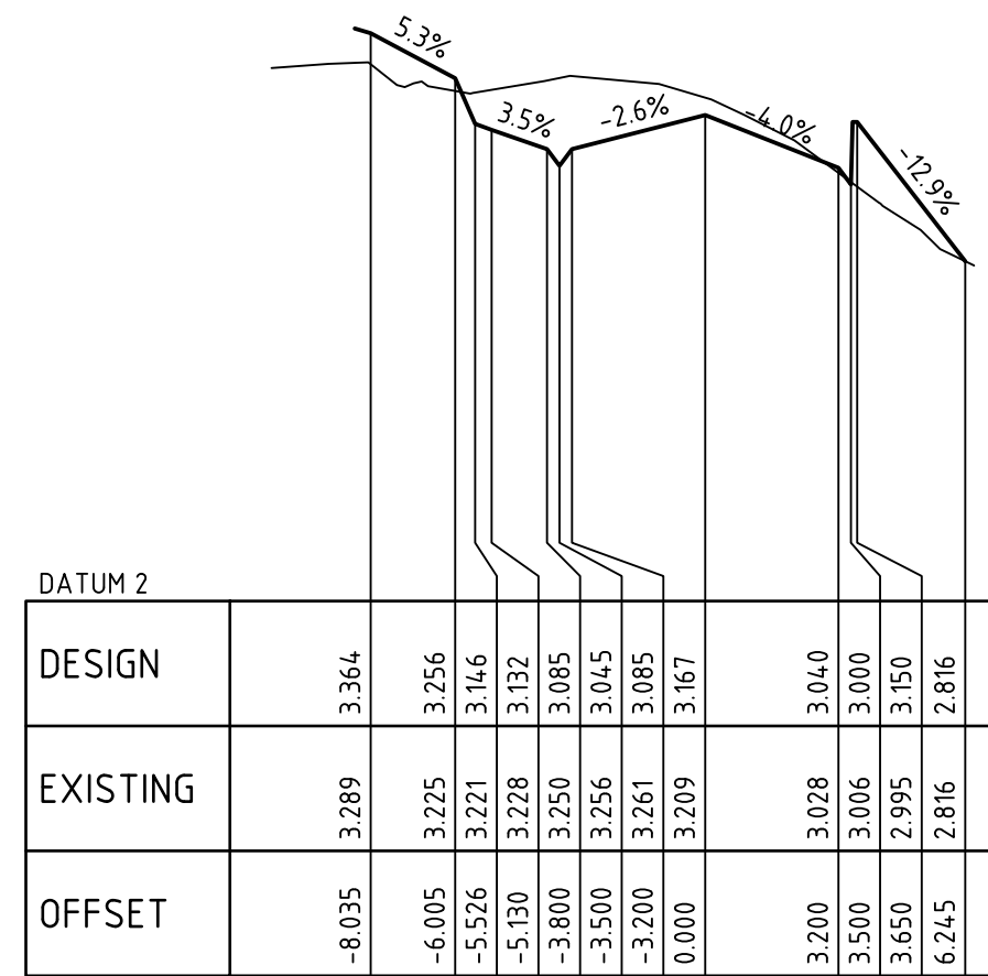
CHAINAGE 20.000
