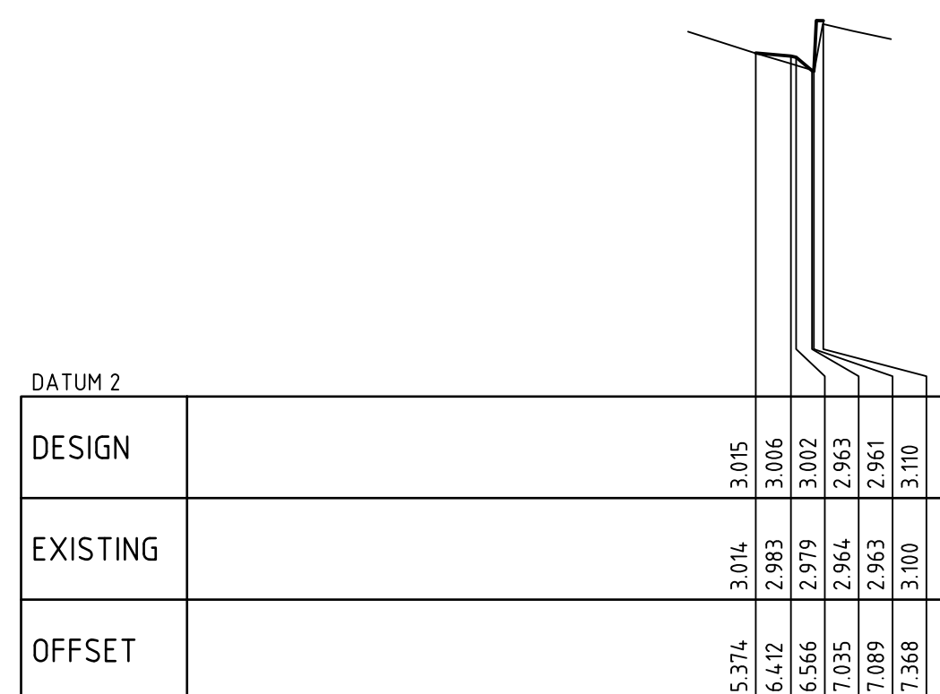
CHAINAGE 6.000
