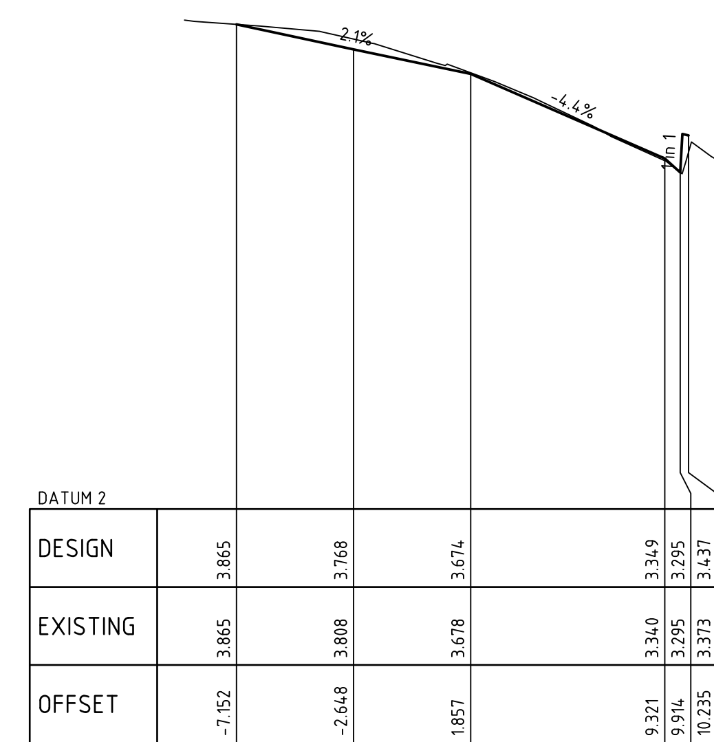
CHAINAGE 200.000
