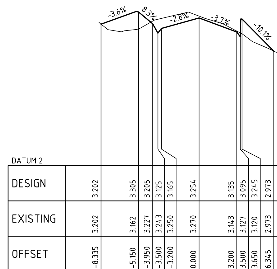
CHAINAGE 60.000
