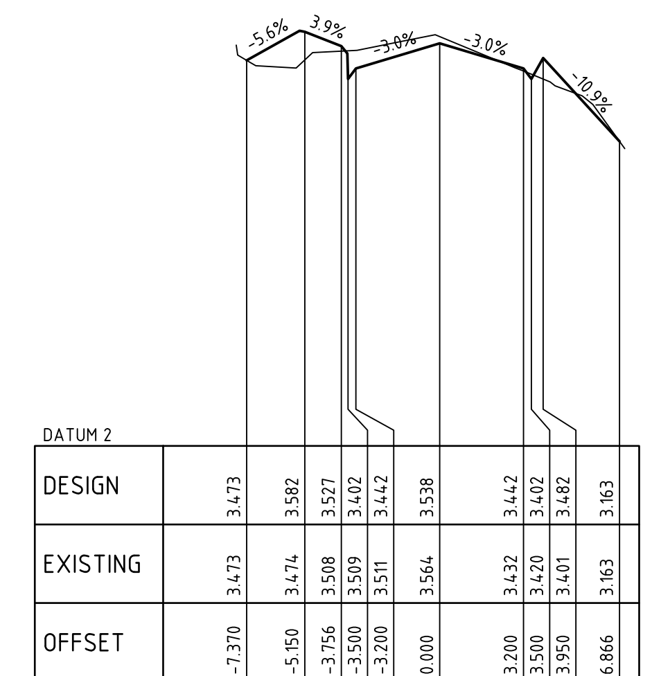
CHAINAGE 240.000
