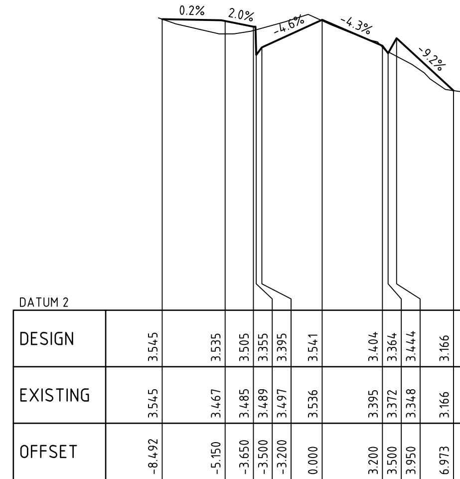
CHAINAGE 140.000
