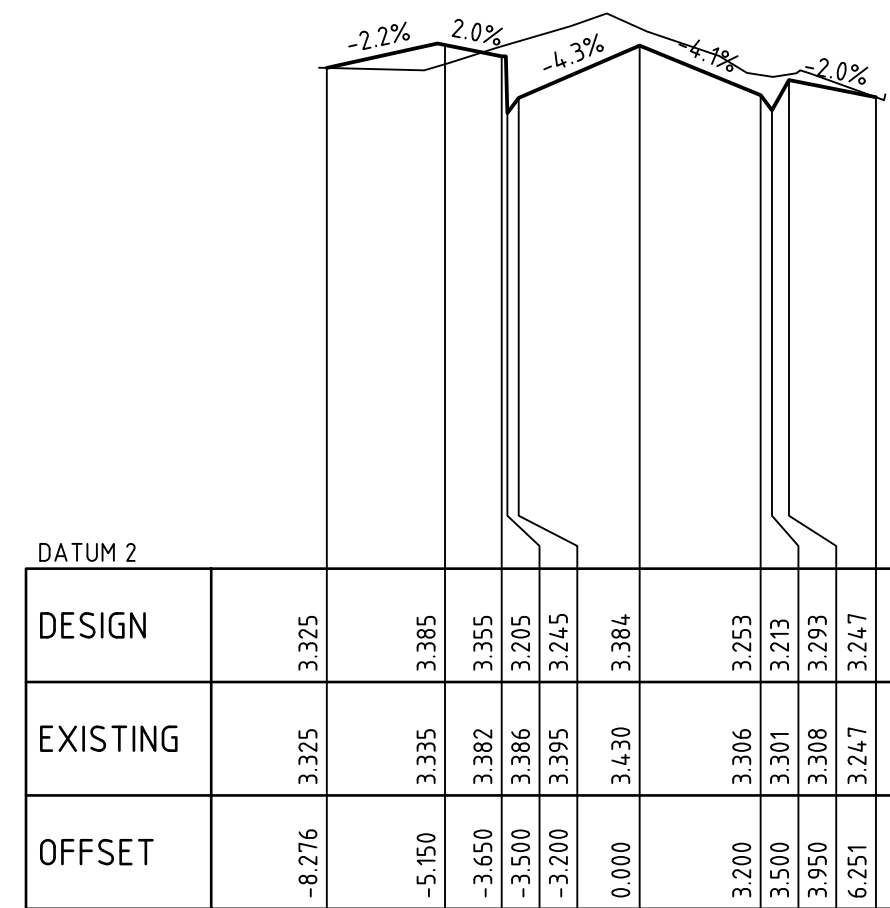
CHAINAGE 100.000
