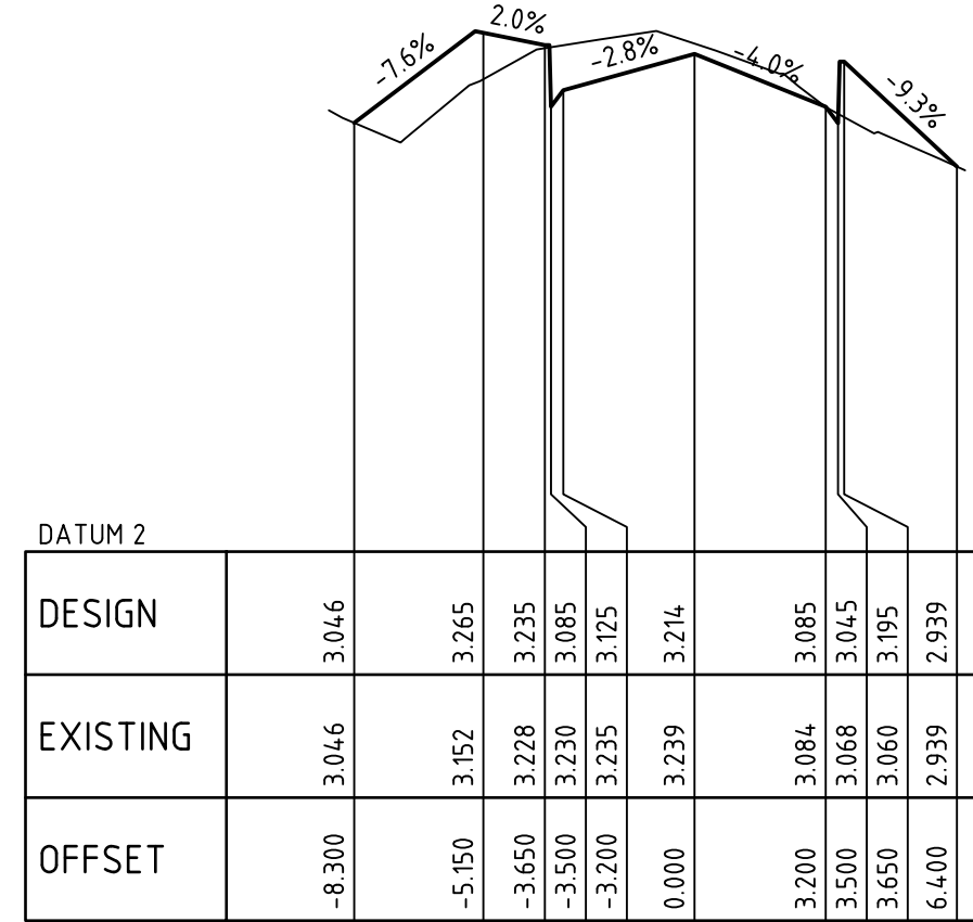
CHAINAGE 40.000
