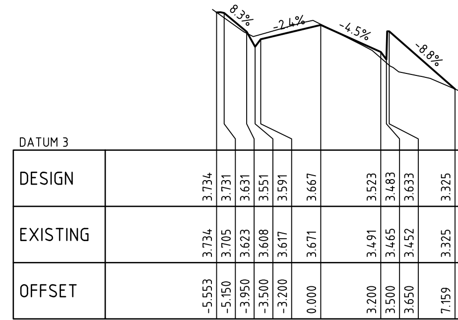
CHAINAGE 160.000
