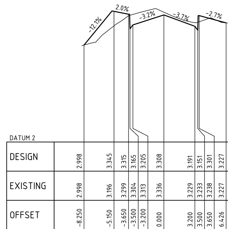
CHAINAGE 80.000
