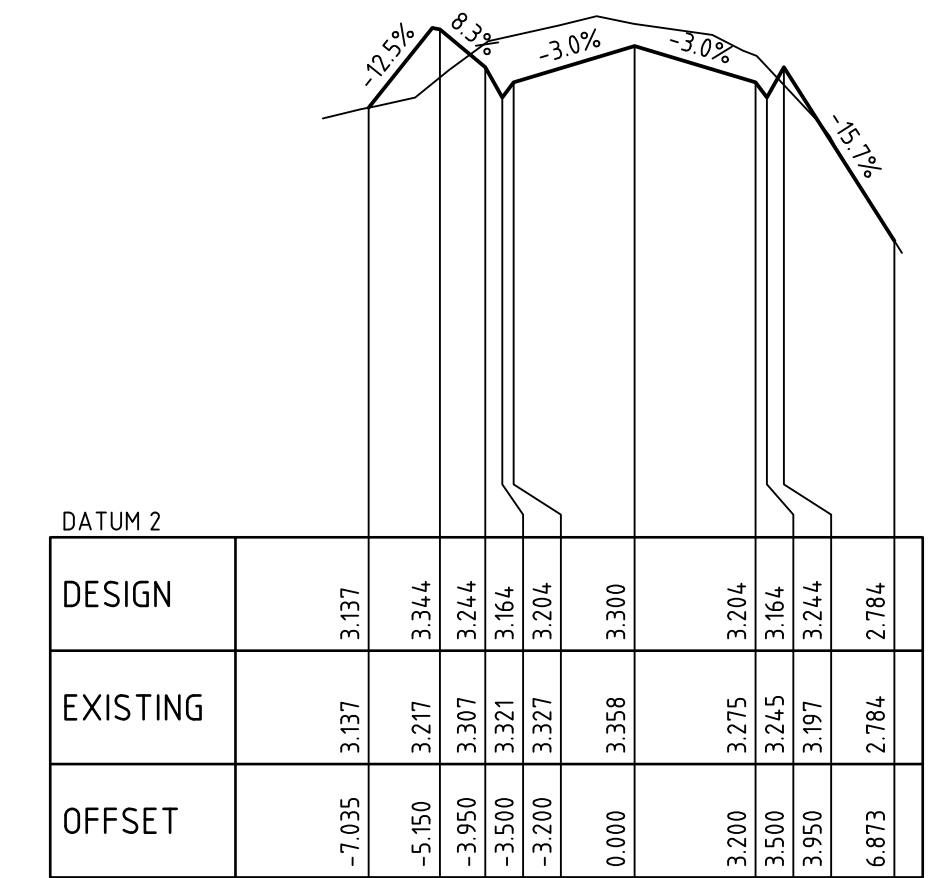
CHAINAGE 280.000
