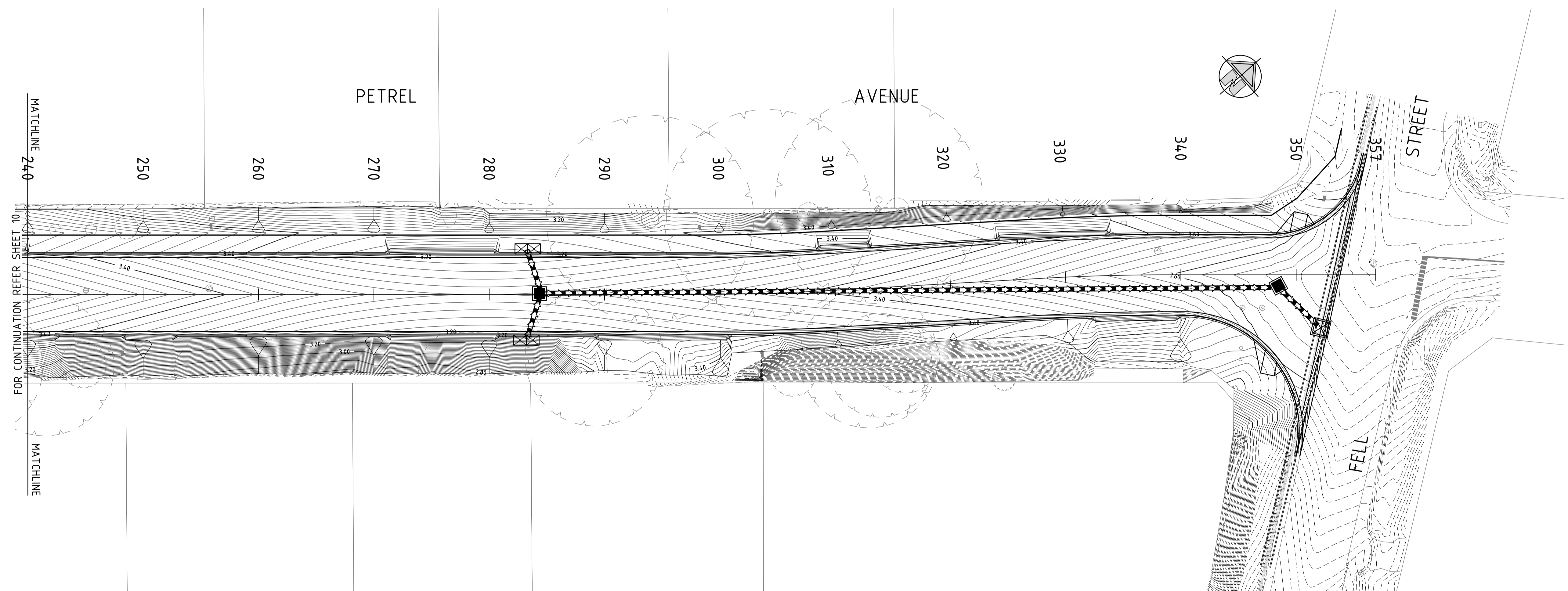
PLAN SCALE: 1:200
